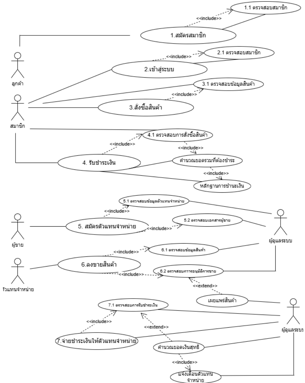
Use case Diagram ระบบขายสินค้ามือสองออนไลน์ ของบริษัท รีแวร์
